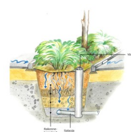
Esimerkkikuvia hulevesien käsittelyrakenteista (Kuvat ylhäältä alas oikealle: Uponor, Rudus ja Ramboll Taru Mäkiranta)
